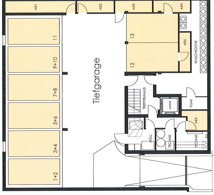
ÜBERSICHTSPLAN Grundriss Untergeschoss
