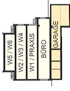
ÜBERSICHTSPLAN Querschnitt
