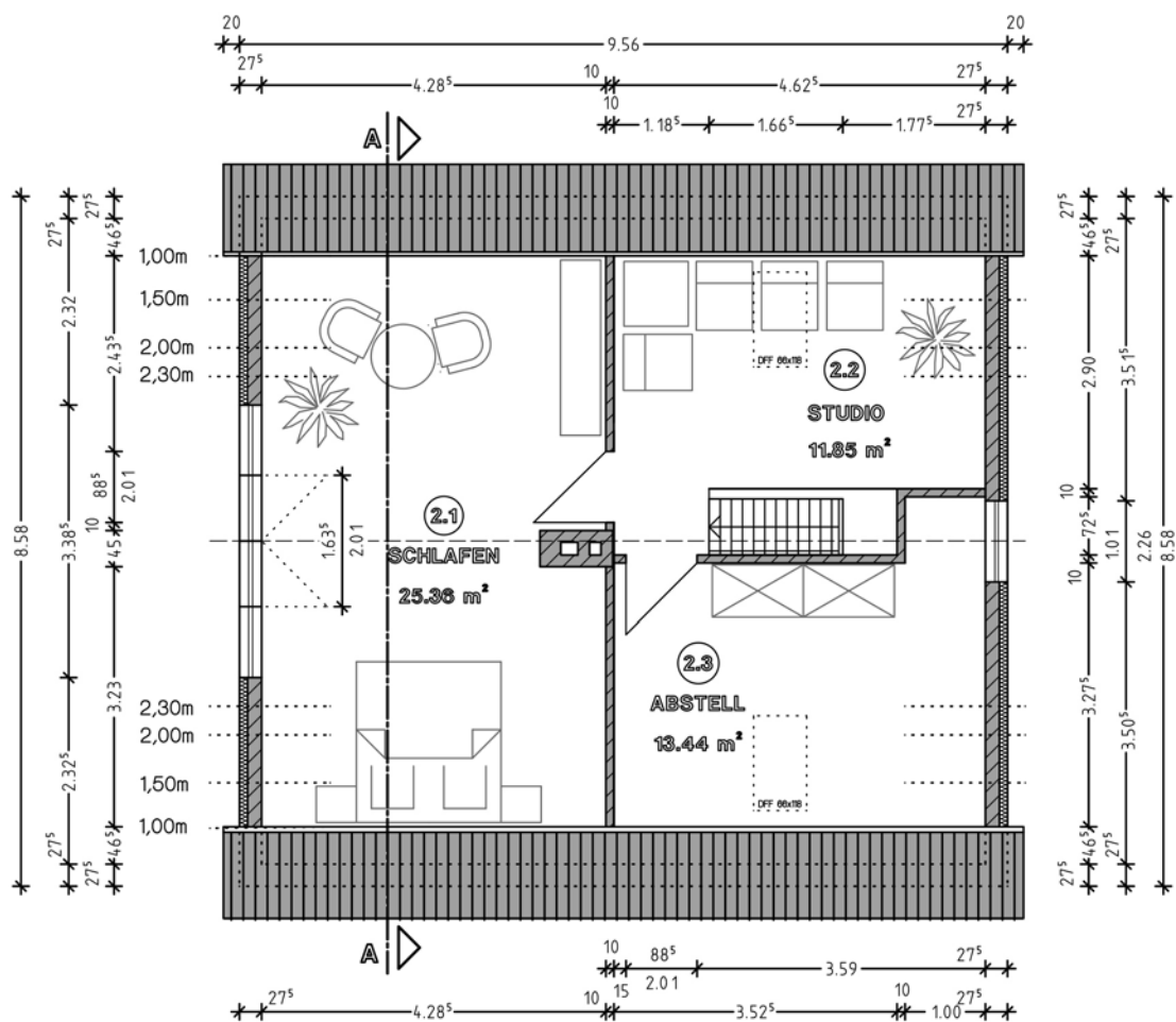
Dachgeschoss M 1: 100
