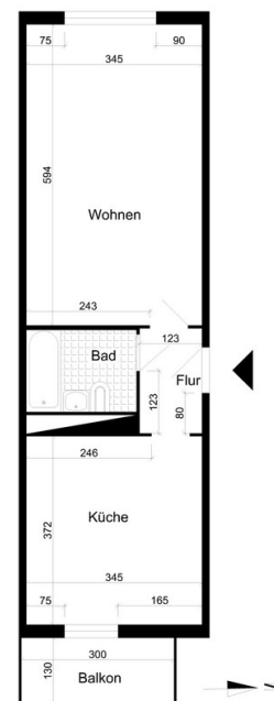
Grundriss
