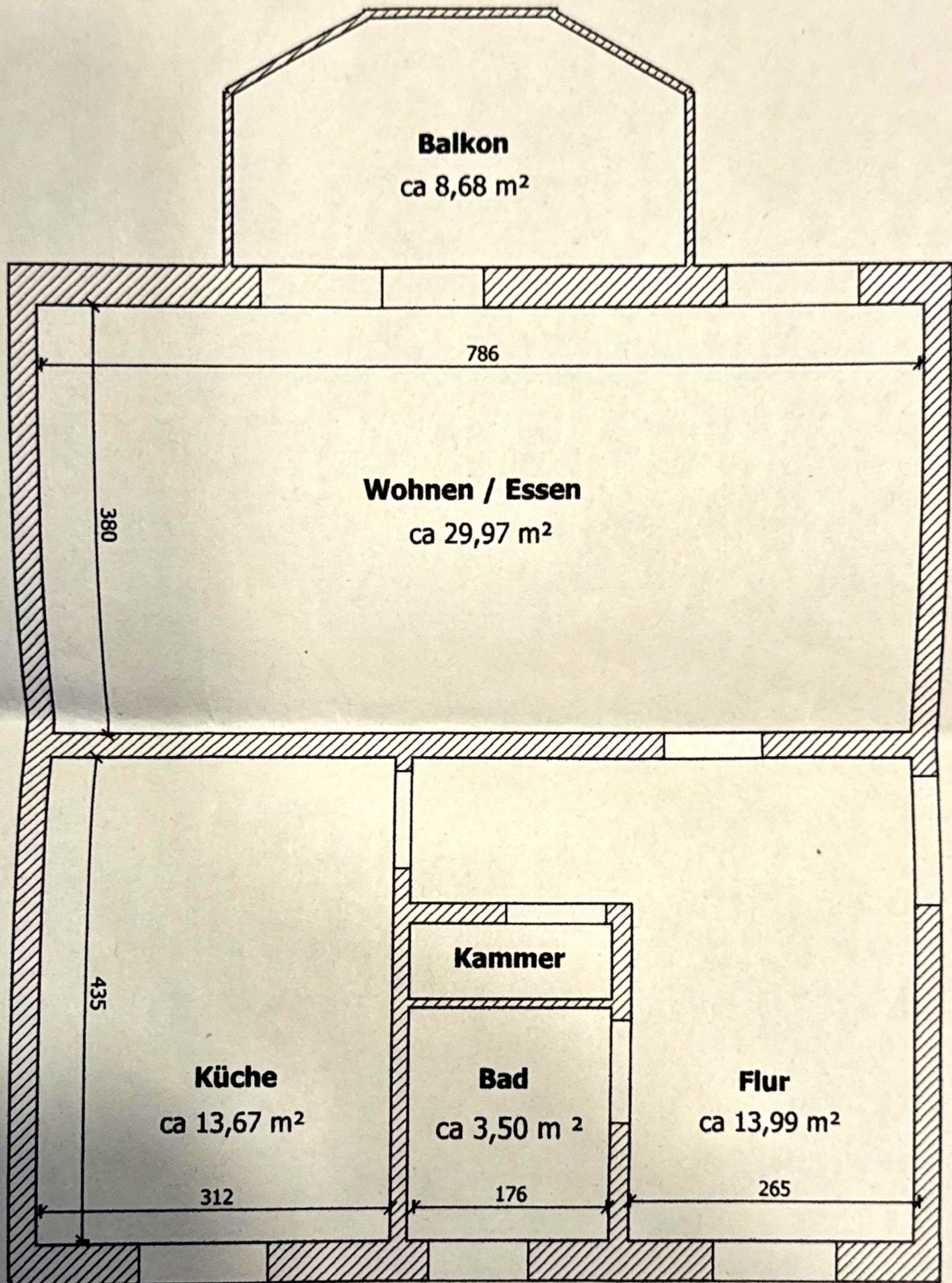
Tröglitz Mittelstr. Wohnung Grundriss Erdgeschoß
