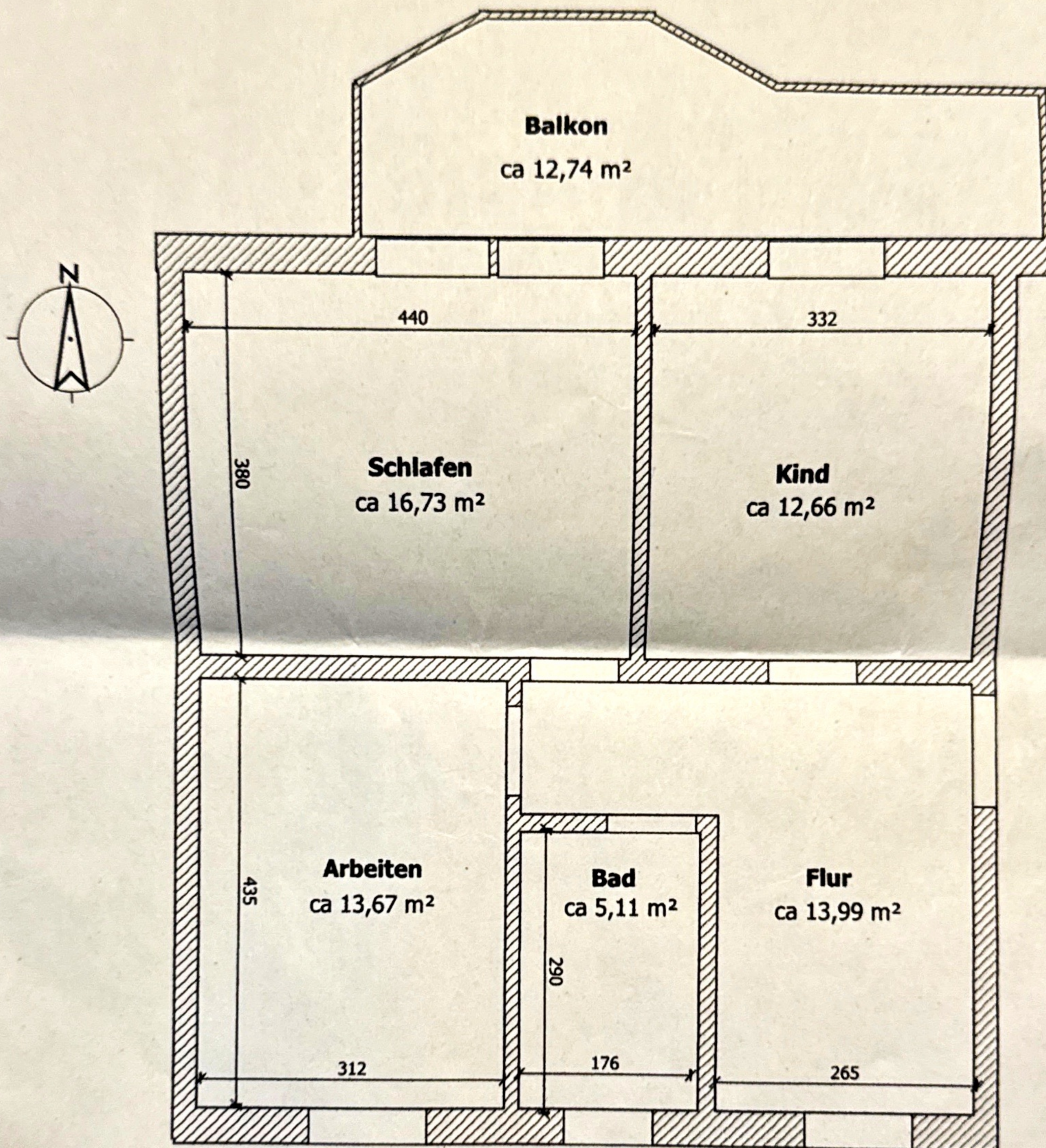
Tröglitz Mittelstr. Wohnung Grundriss Obergeschoß
