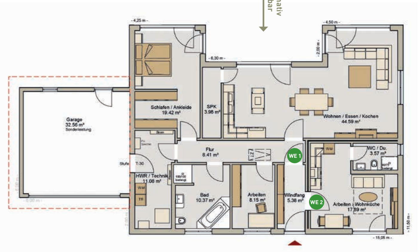
Erdgeschoss
