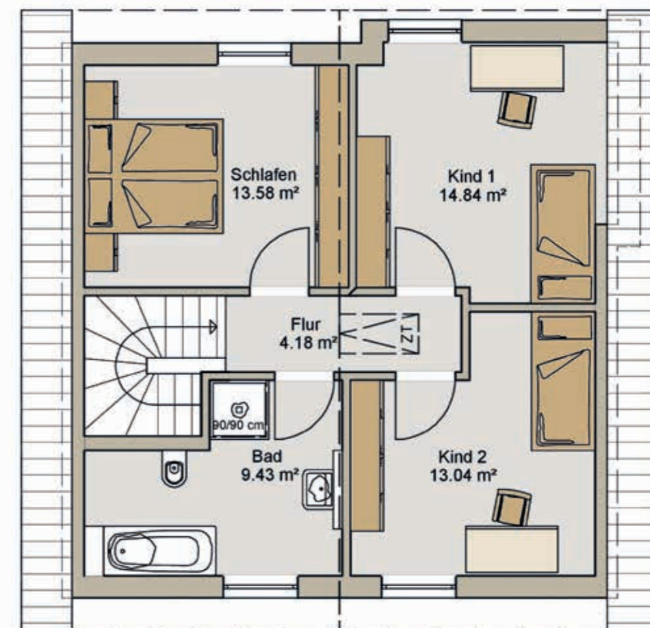
Dachgeschoss
