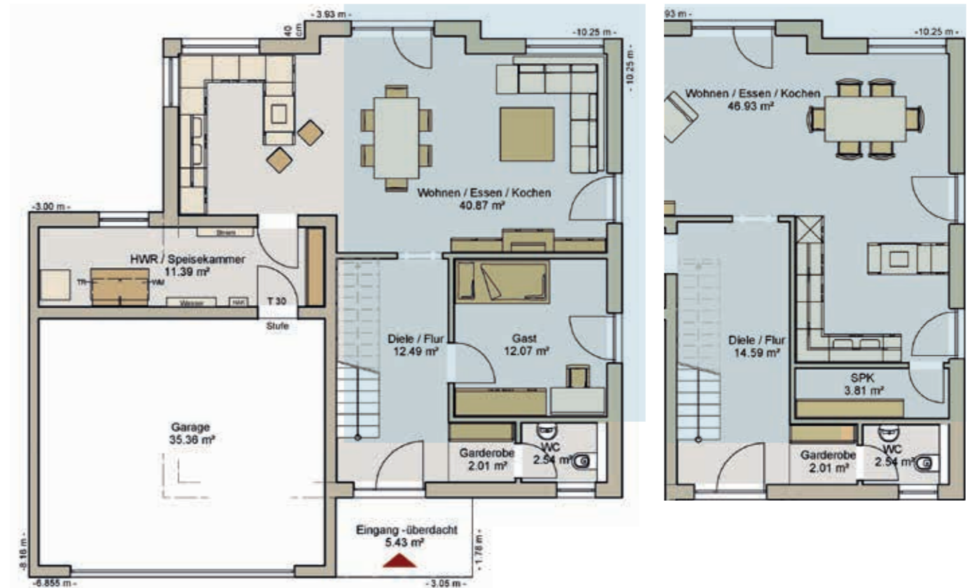
Erdgeschoss
