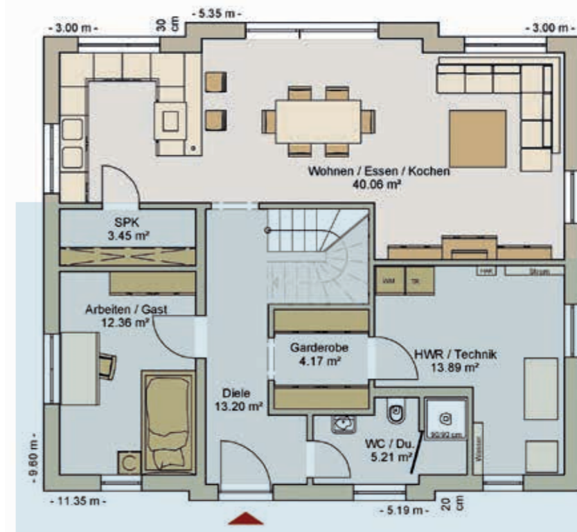
Erdgeschoss
