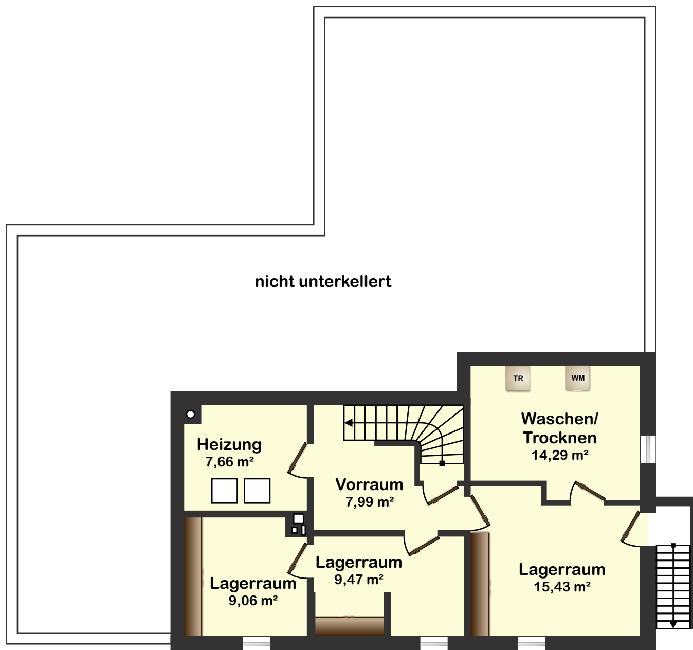
Kellergeschoss
