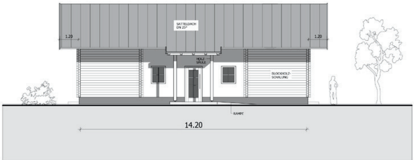
NORDANSICHT M 1/100
