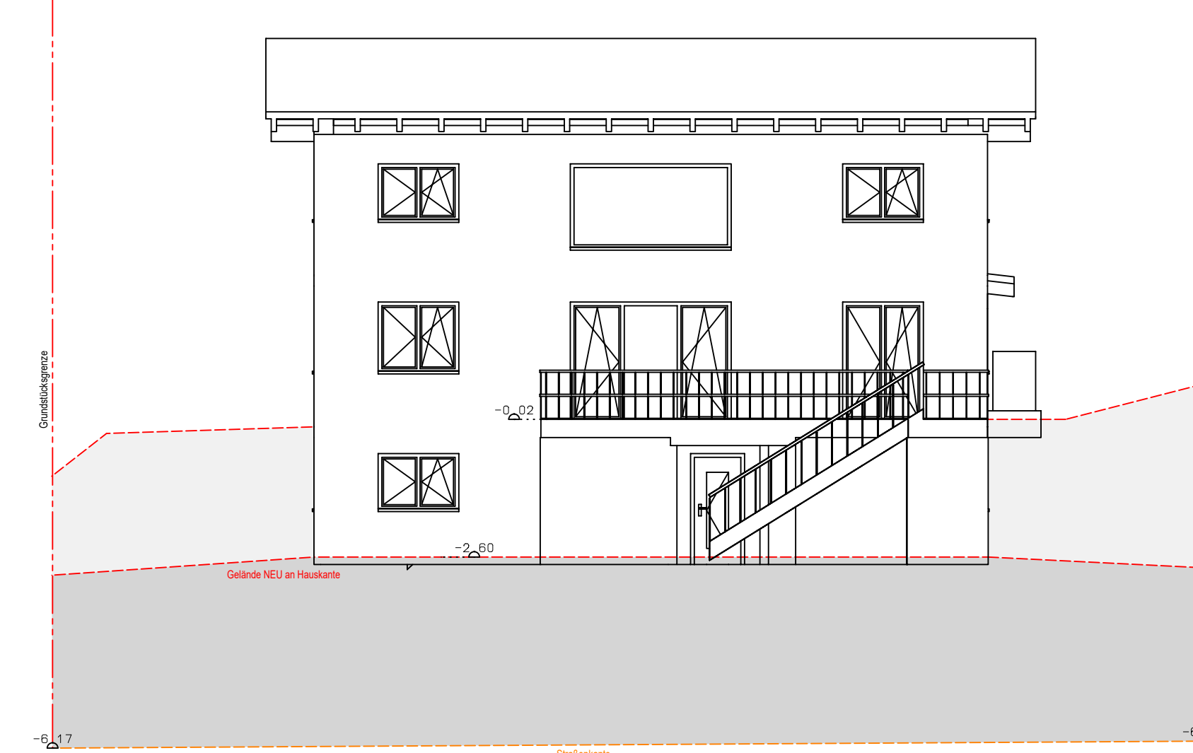
Ansicht Süden
