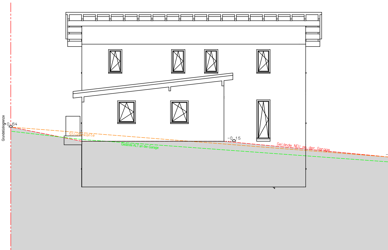
Ansicht Norden
