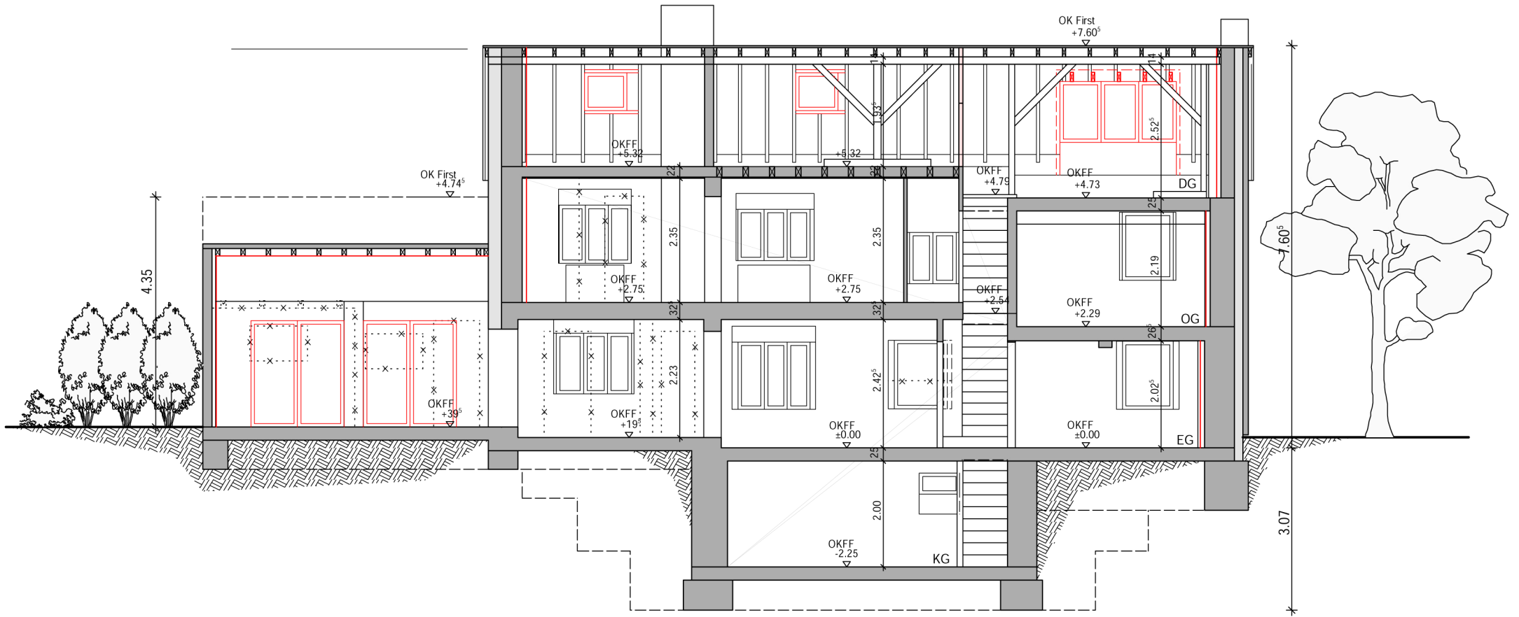
Schnitt B
