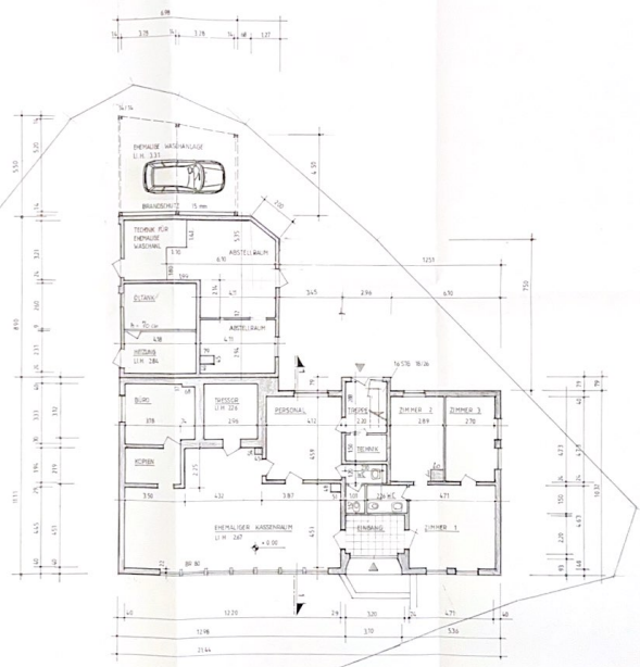
EG-GRUNDRISS 1:100
