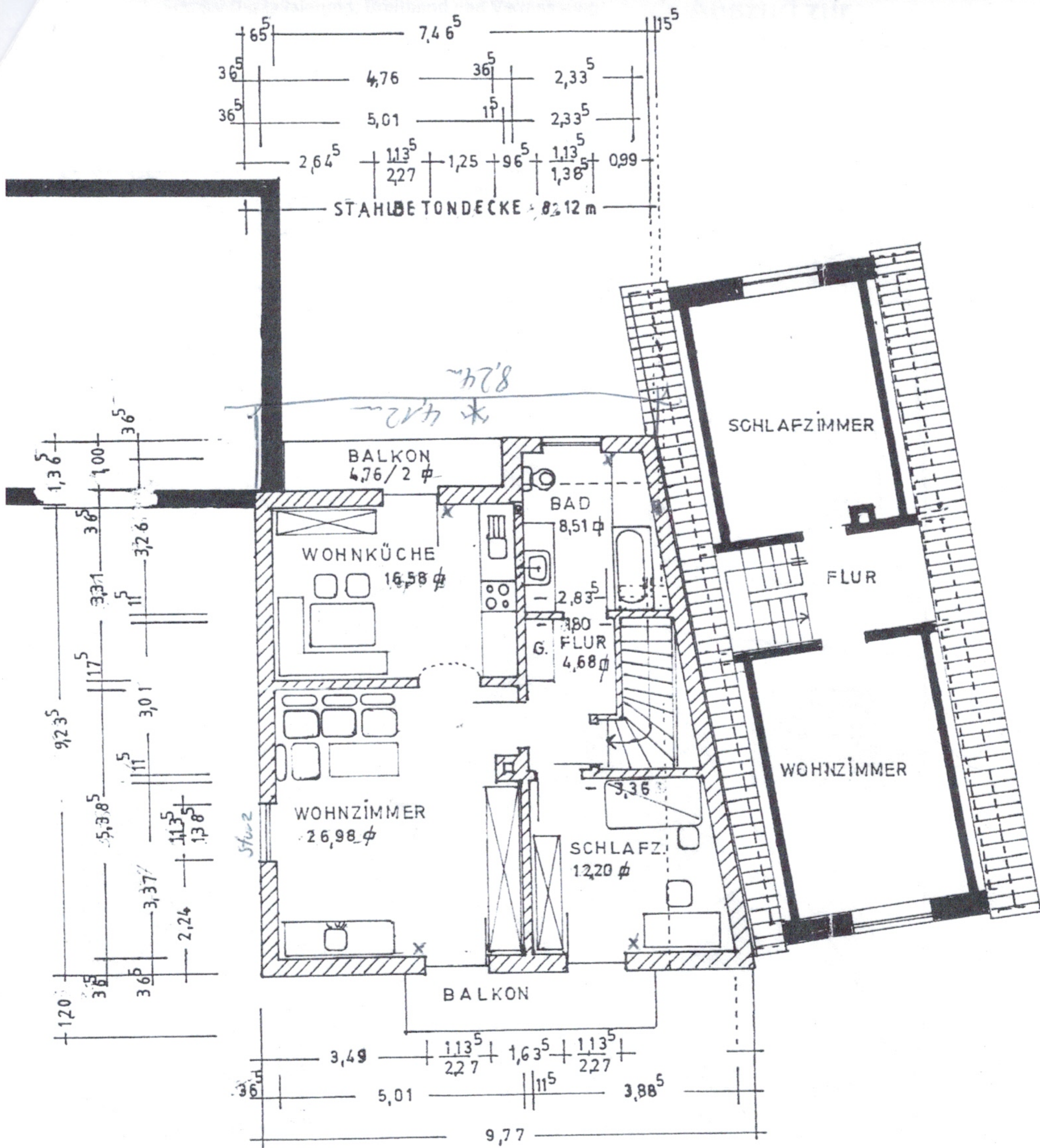
GRUNDRISS OBERGESCHOSS
