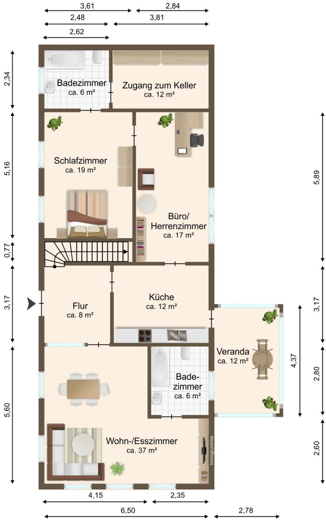
Erdgeschoss
