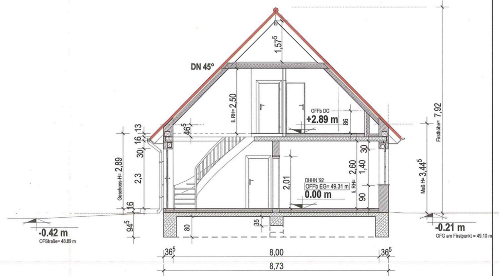
Querschnitt 1:100
