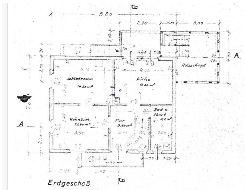
Grundrisse EG
