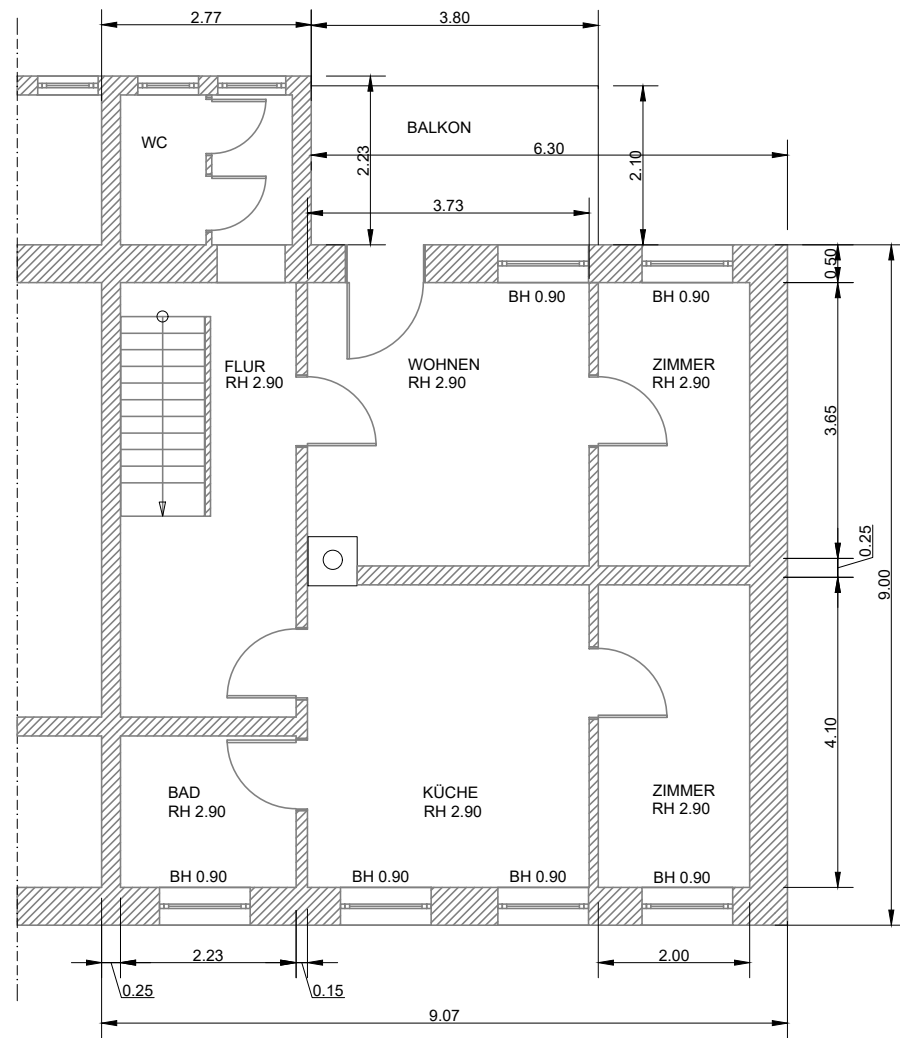
OBERGESCHOSS M 1:100
