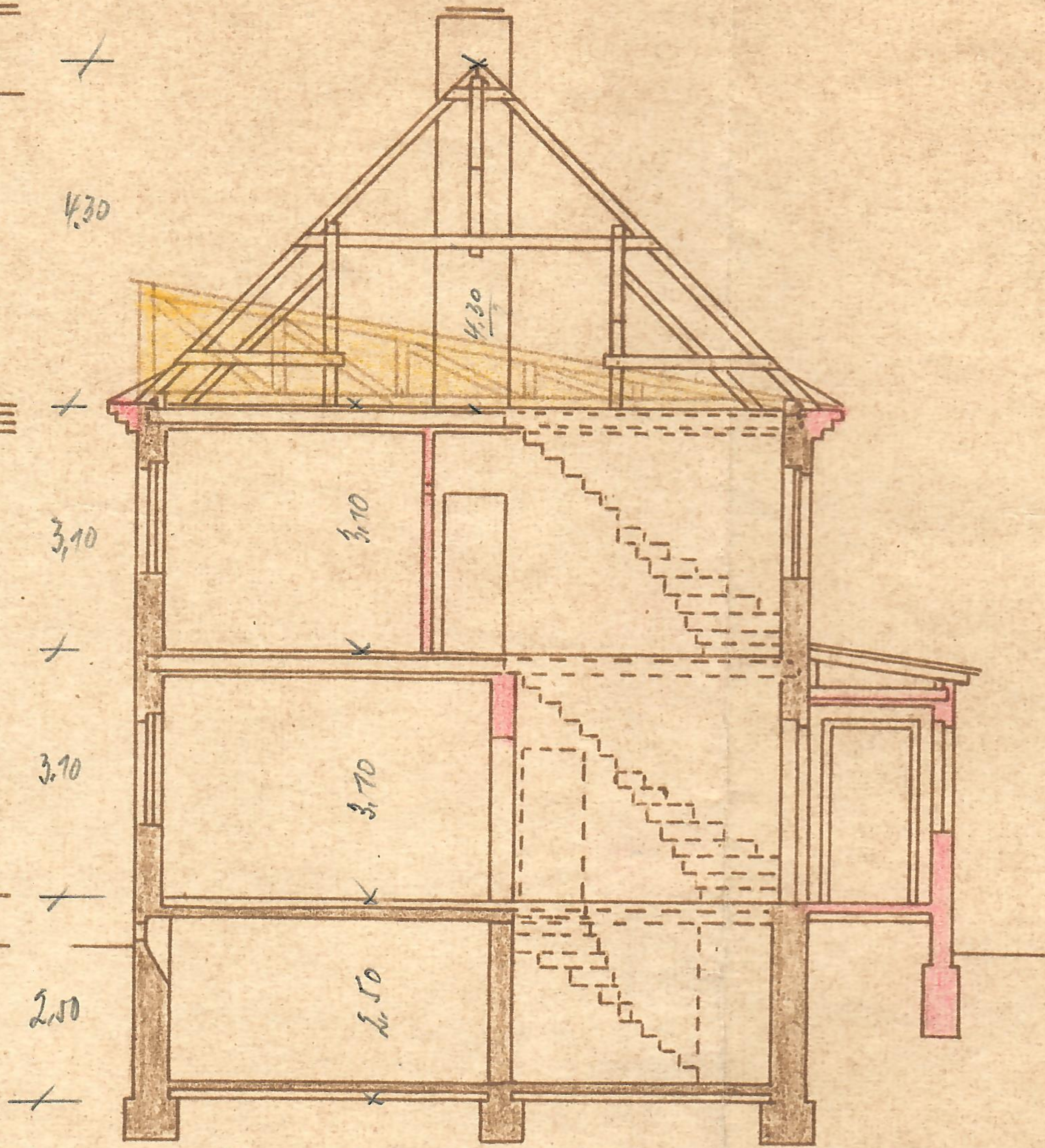
Schnitt A-B
