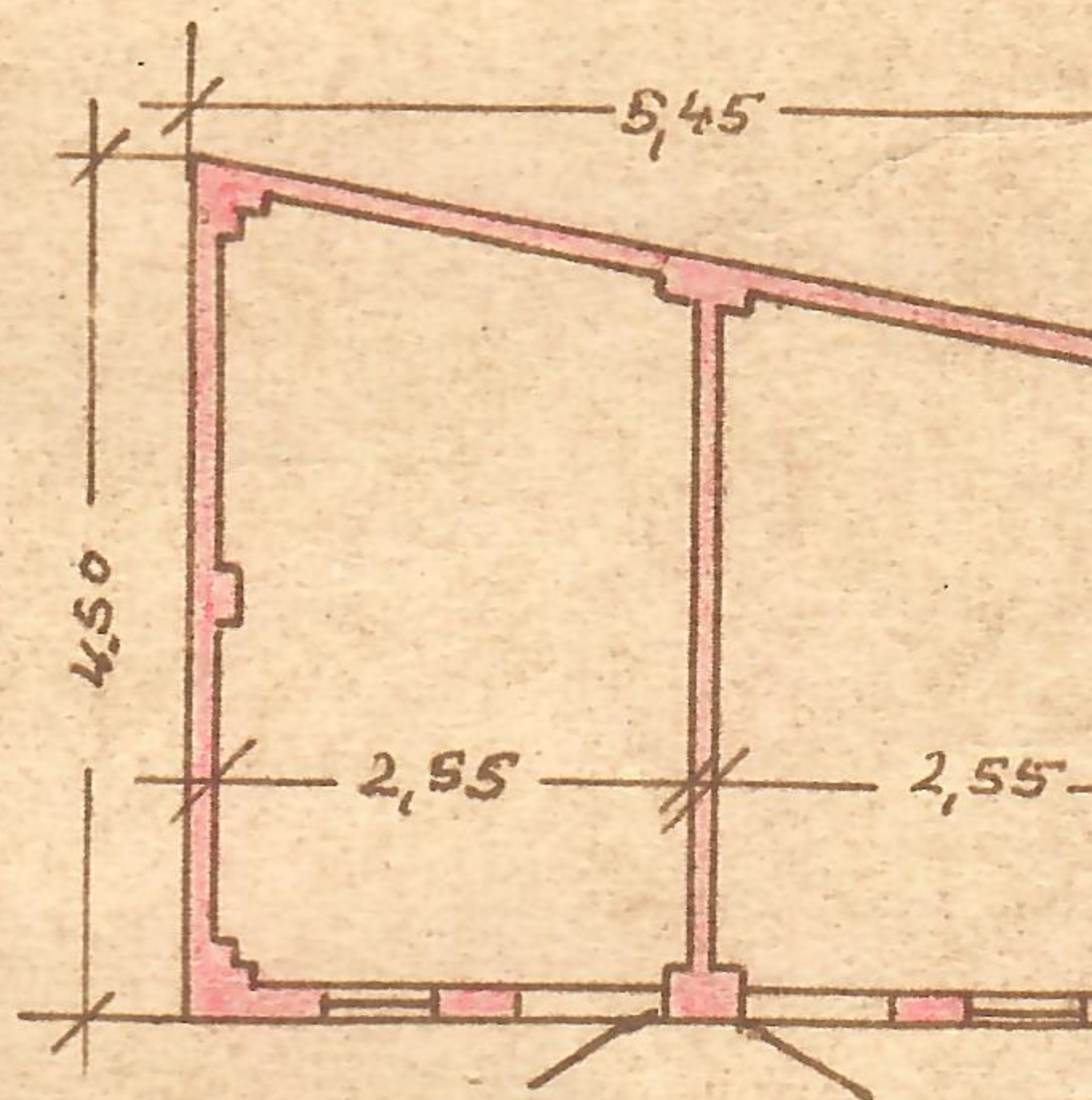
Schuppen Stall
