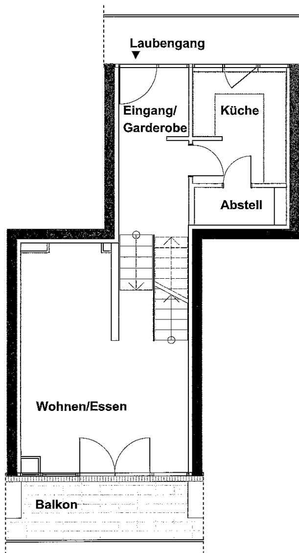
Eingangsgeschoss
