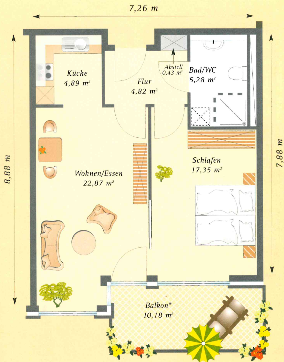
Erdgeschoß
