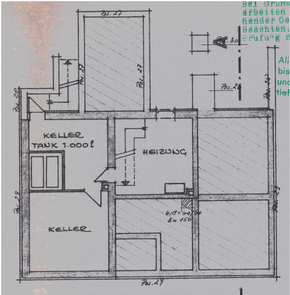
Grundrisszeichnung Kellergeschoss
