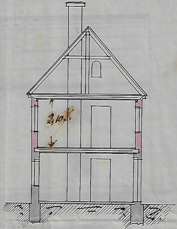
Schnitt a-b.
