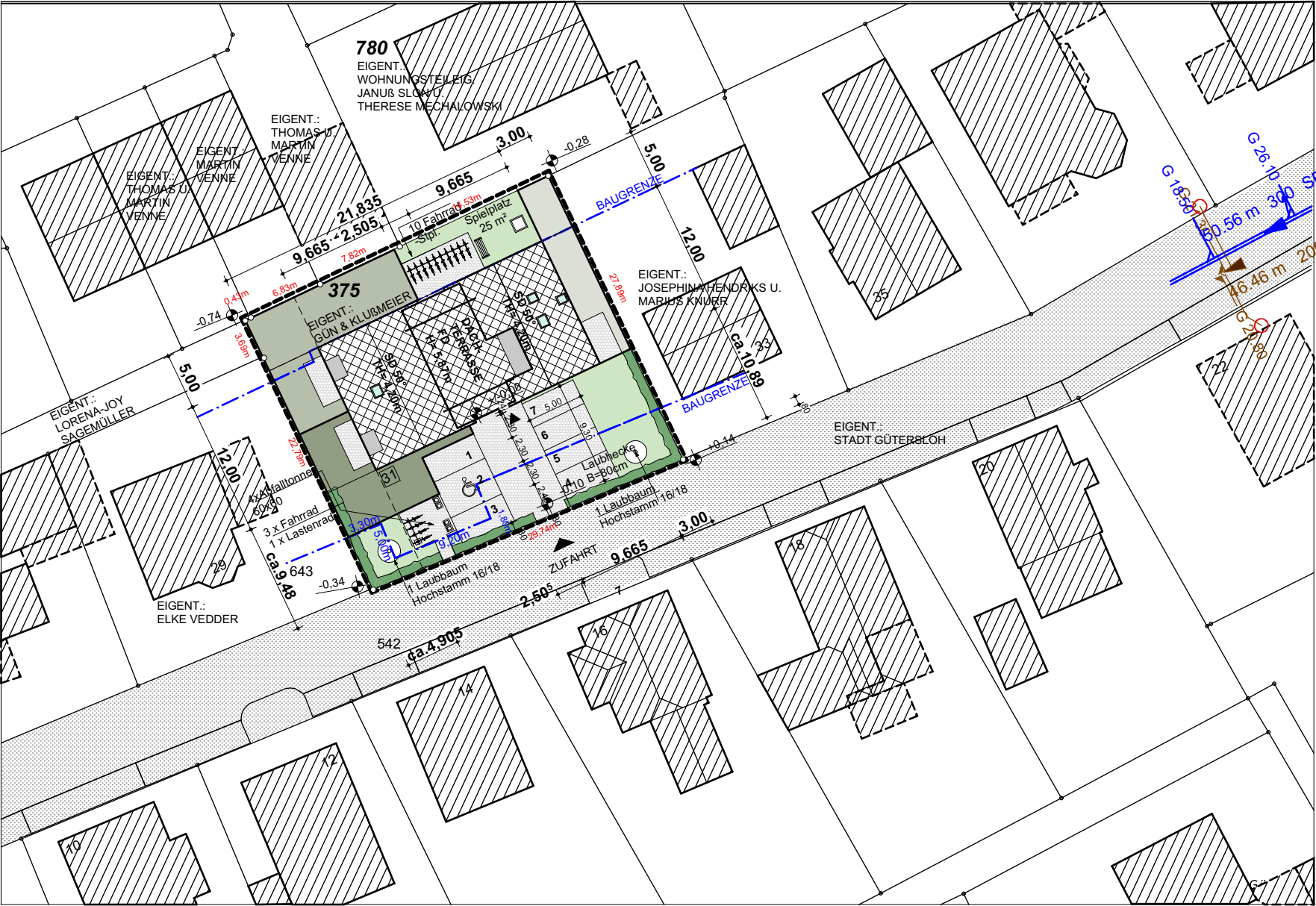
LAGEPLAN M.1:500
