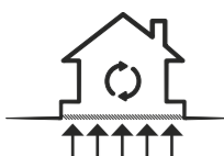
aufsteigendes Radon
