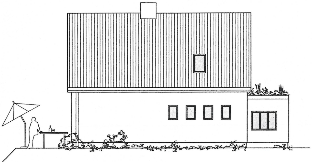
Ansicht Nord-West
