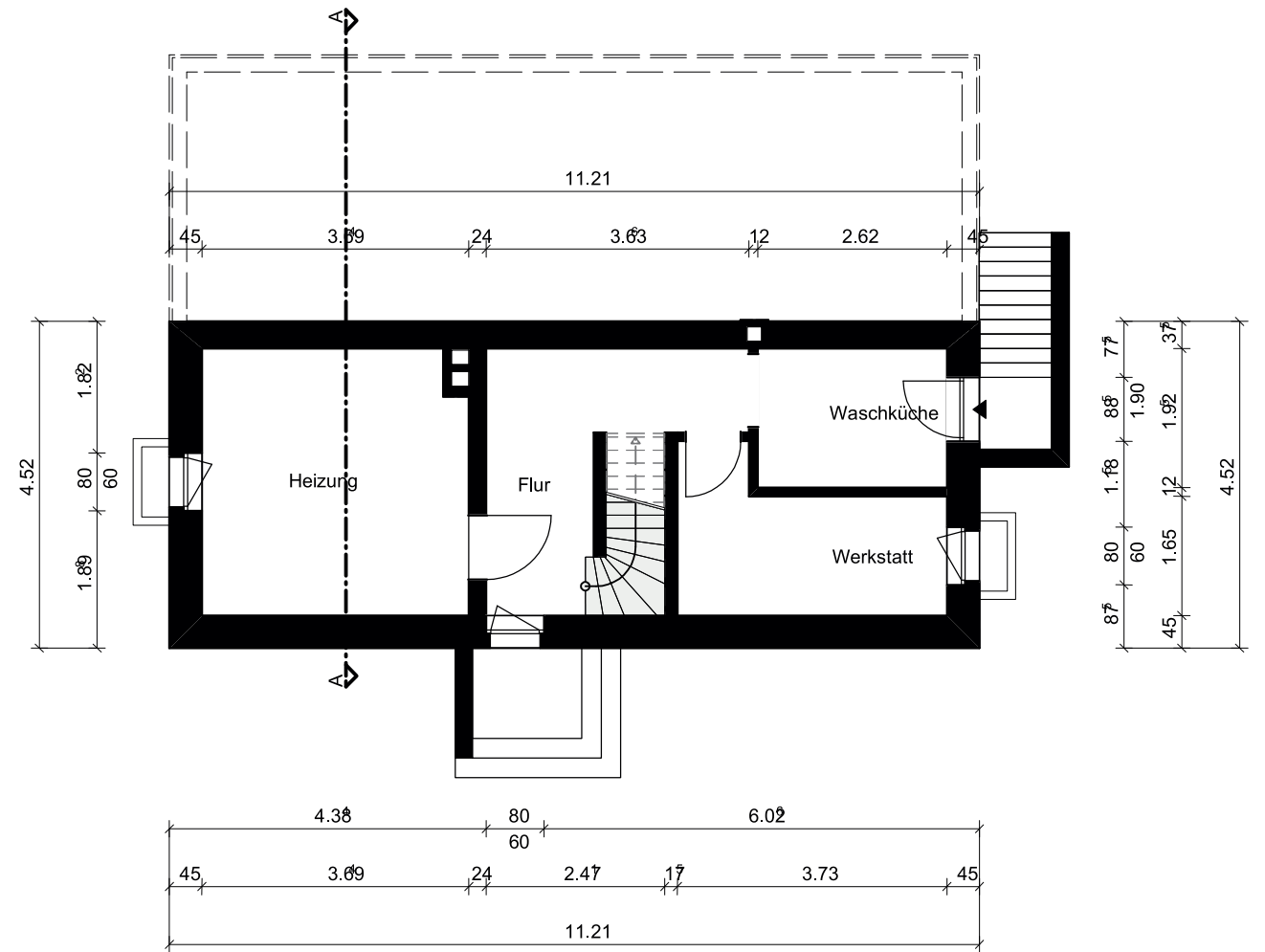
KELLERGESCHOSS
