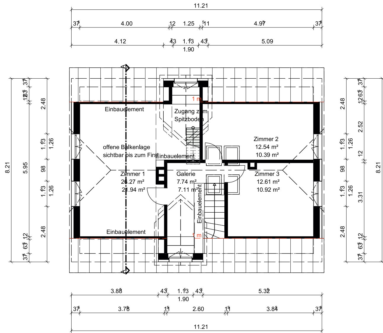
DACHGESCHOSS
