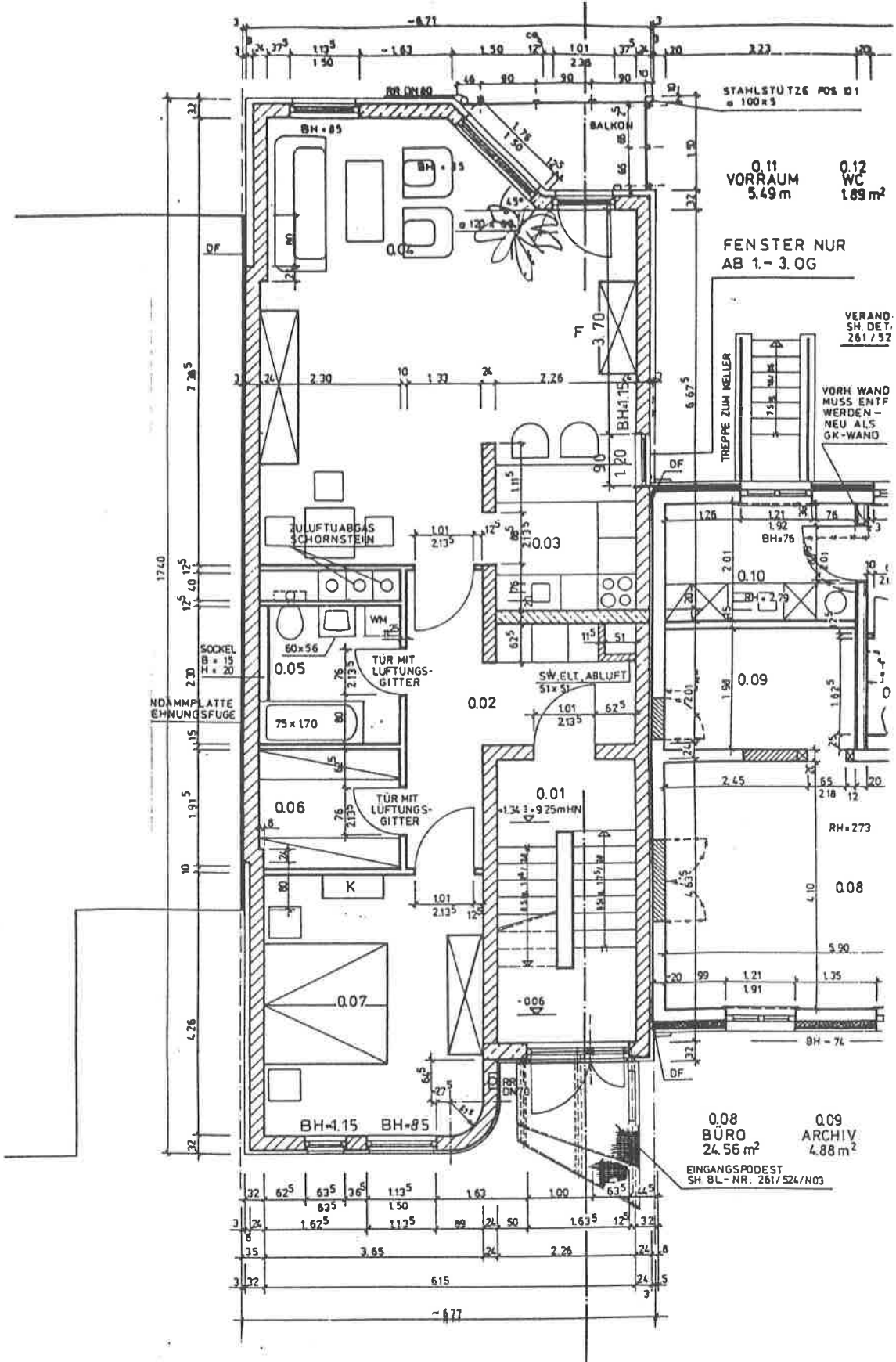
JUNGFERNSTIEG 4 GRUNDRISS EG - 2.0G M 1:100
