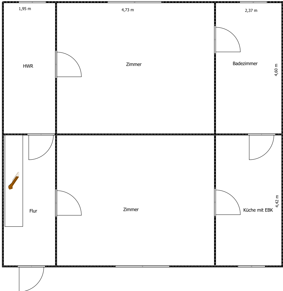
Grundriss: EG
