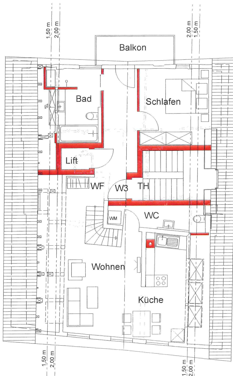
2.OBERGESCHOSS / 69 m 2
