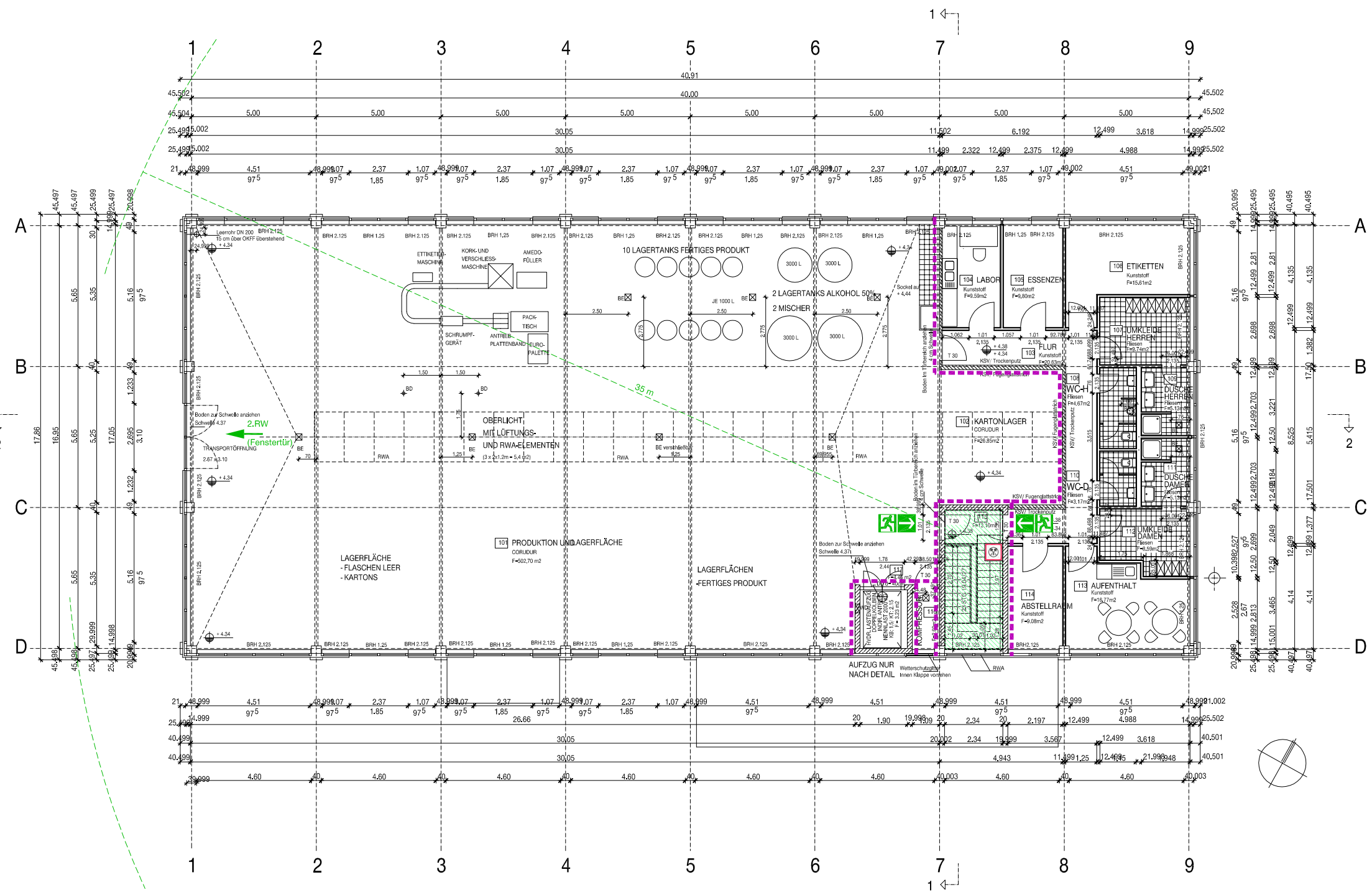
GRUNDRISS OBERGESCHOSS
