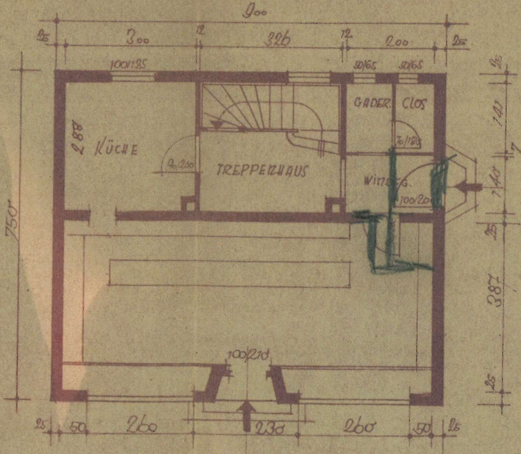
ERDGESCHOSSGRUNDRISS
