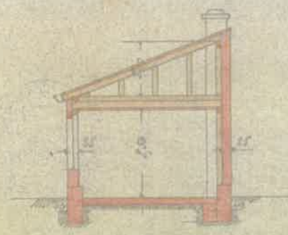
Querschnitt
