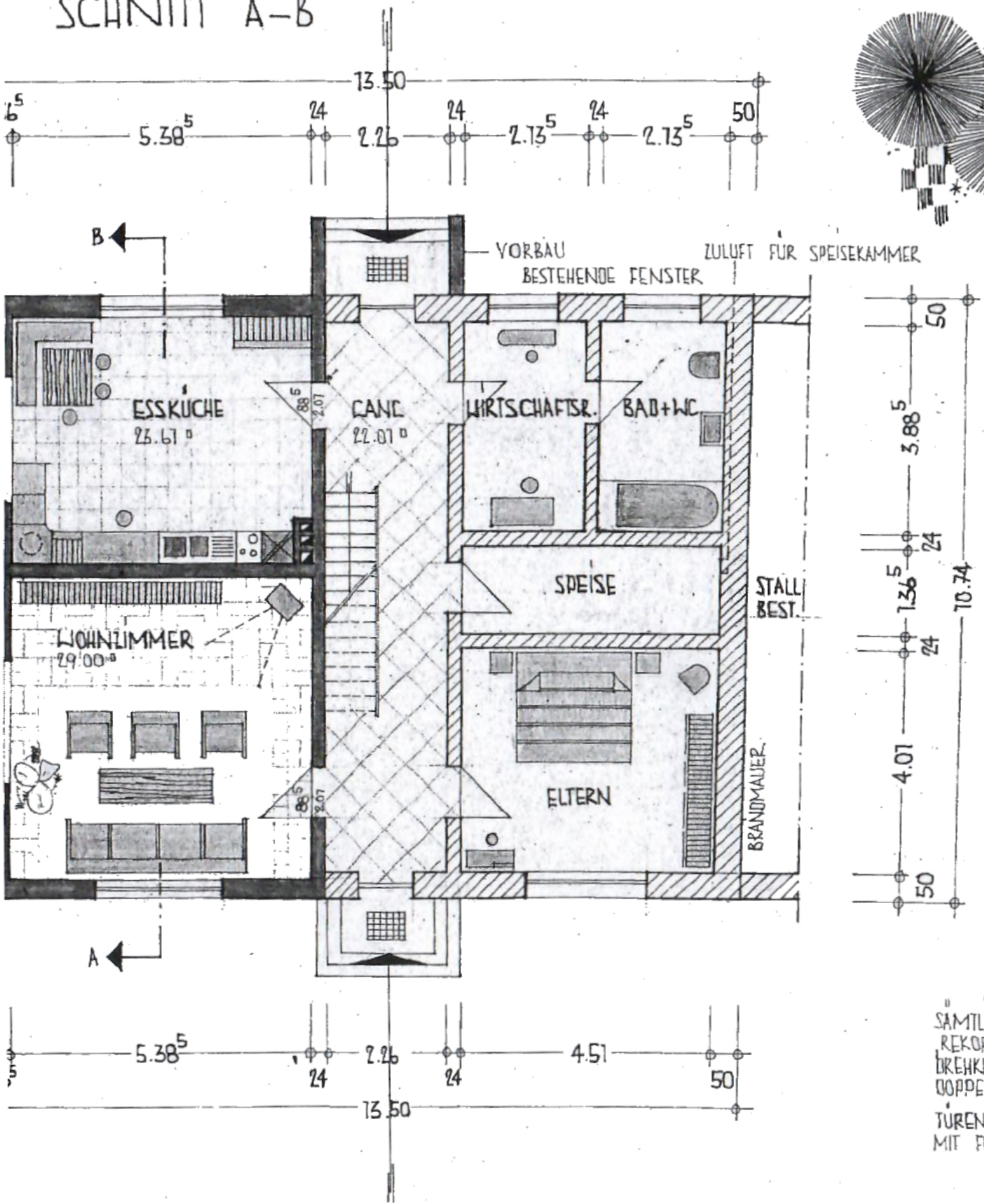
ERDGESCHOSS
