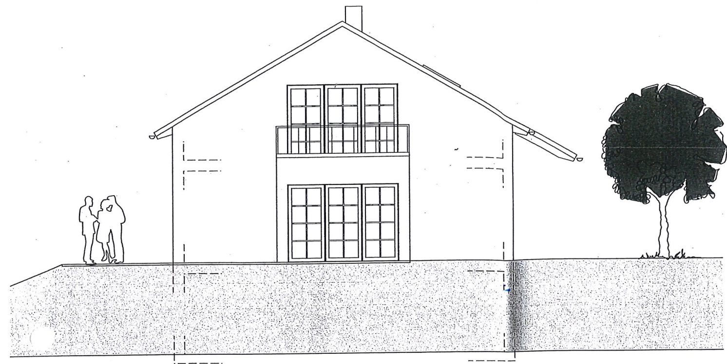
Ansicht Südwest
