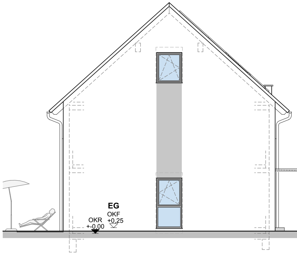
Giebelansicht
