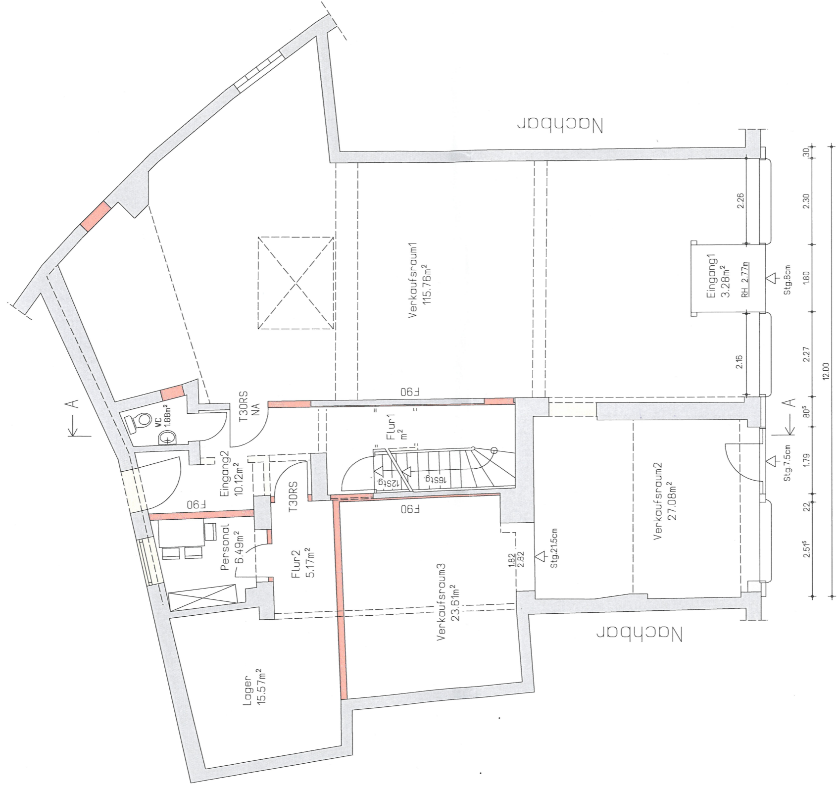
ERDGESCHOSS VORABZUG 20.11.2014 1:100
