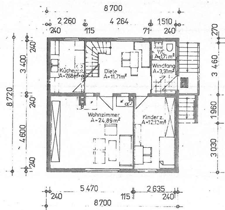
Erdgeschoss
