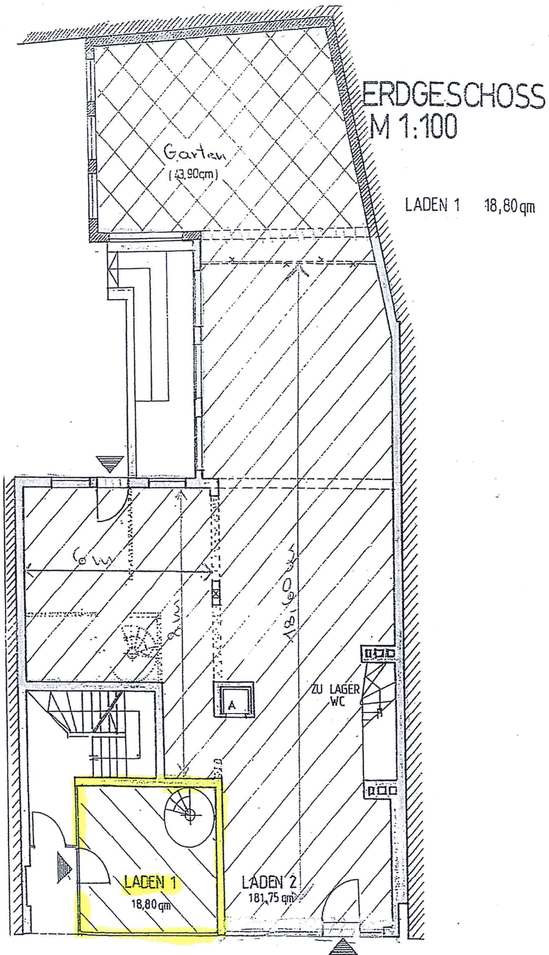
Grundriss Erdgeschoss Laden 1
