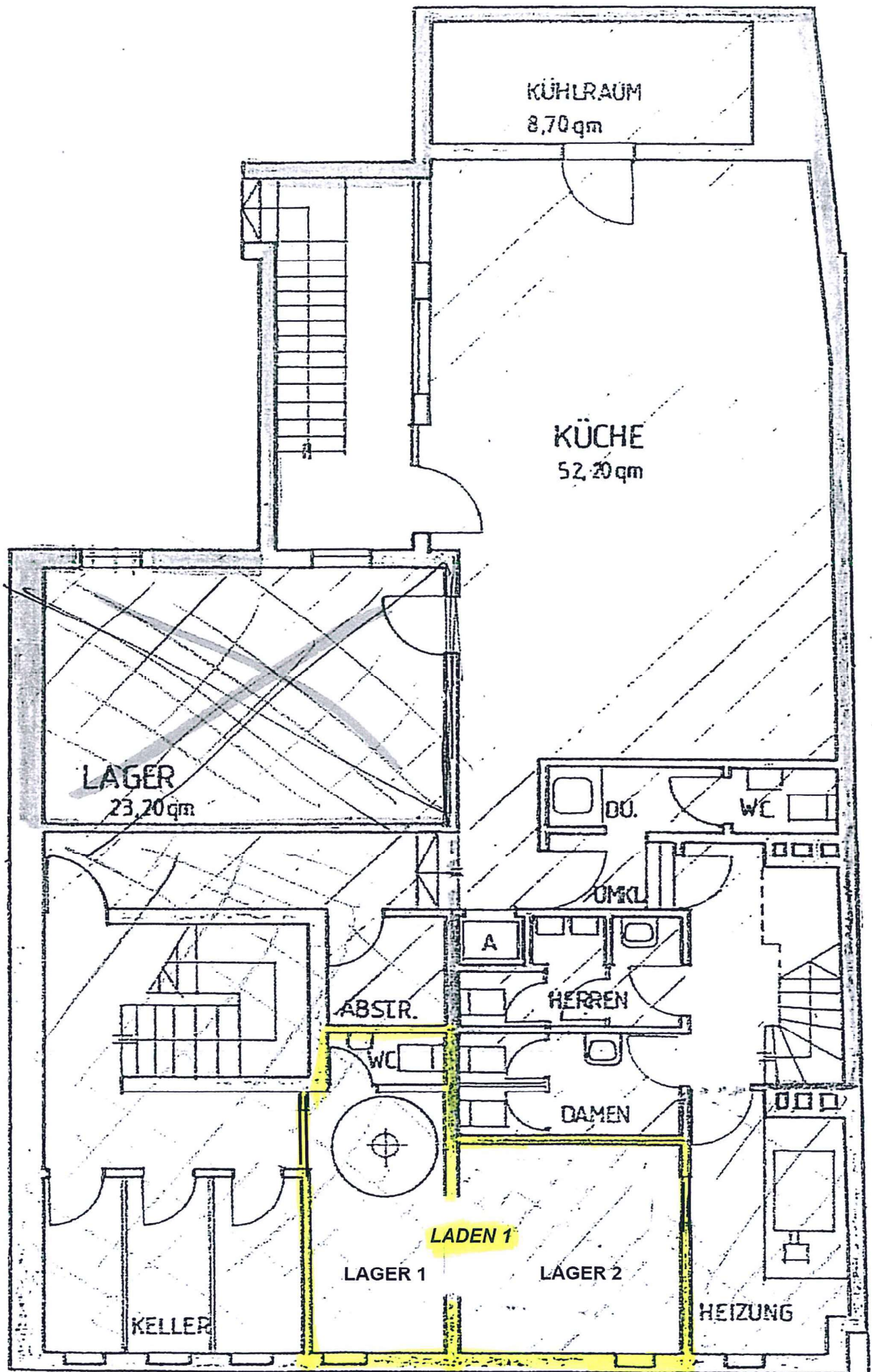
Grundriss Kellergeschoss Laden 1
