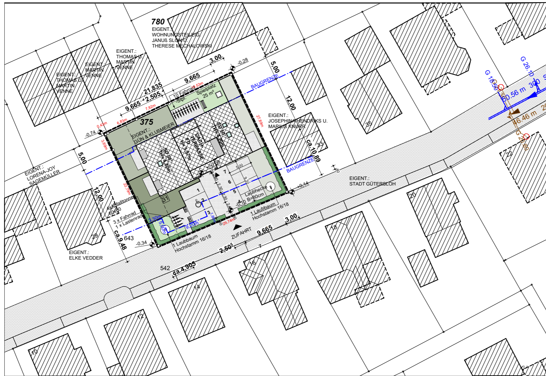
LAGEPLAN M.1:500
