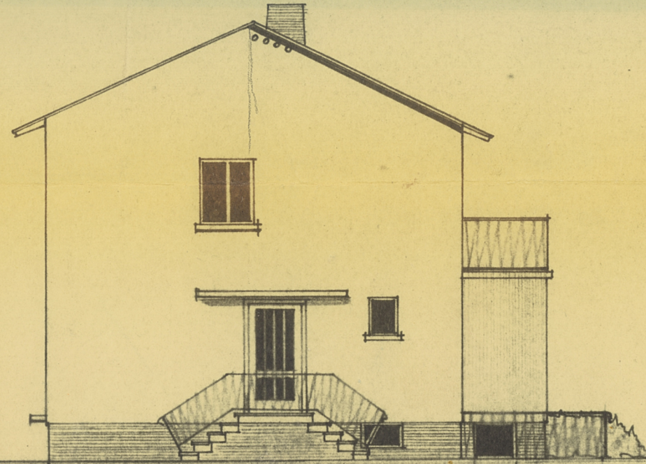
SEITENANSICHT (NORD)
