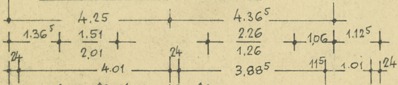
STRASSENANSICHT
