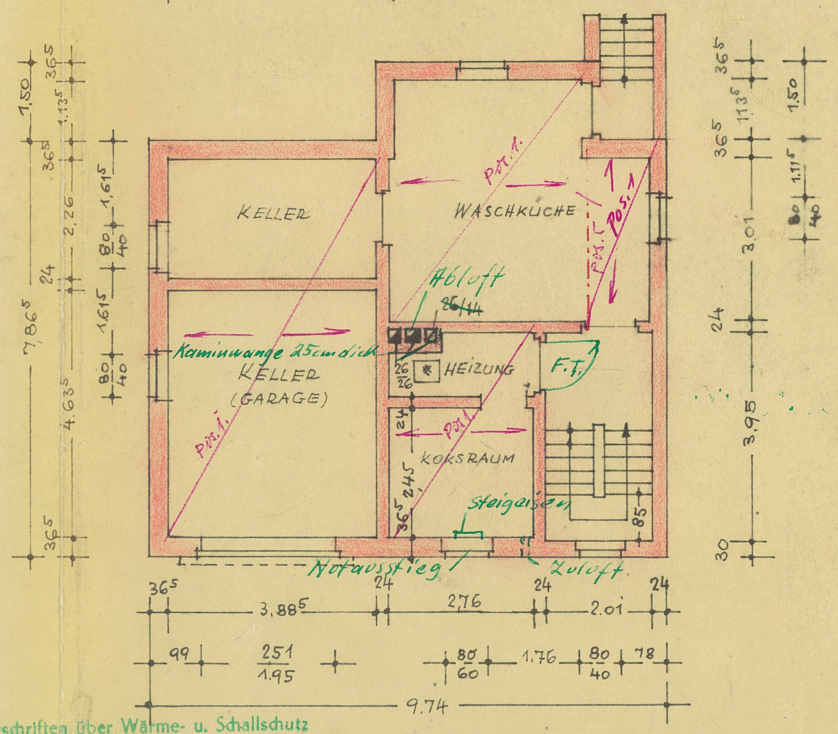
KELLERGESCHOSS
