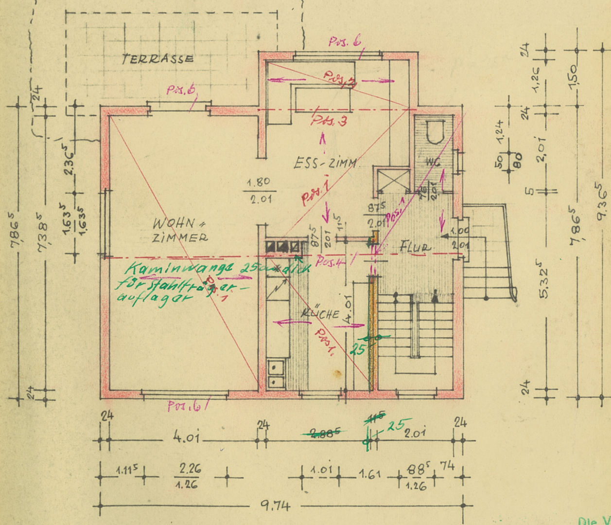
ERDGESCHOSS
