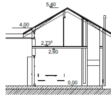
B Schnitt B-B 1:100
