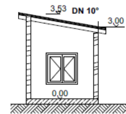
C Schnitt C-C 1:100
