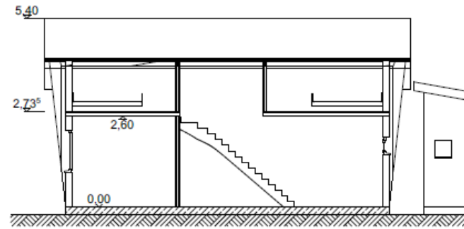
A Schnitt A-A 1:100
