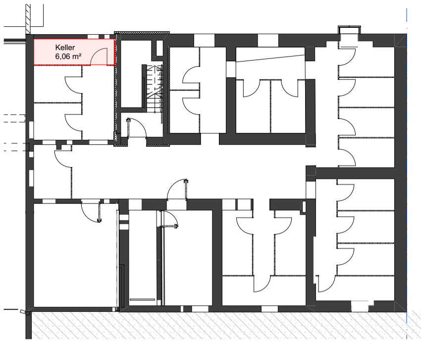
Mieterkeller Maßstab 1:200
