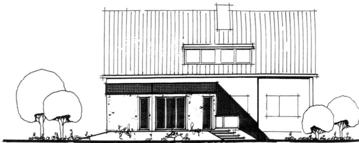
OSTANSICHT
