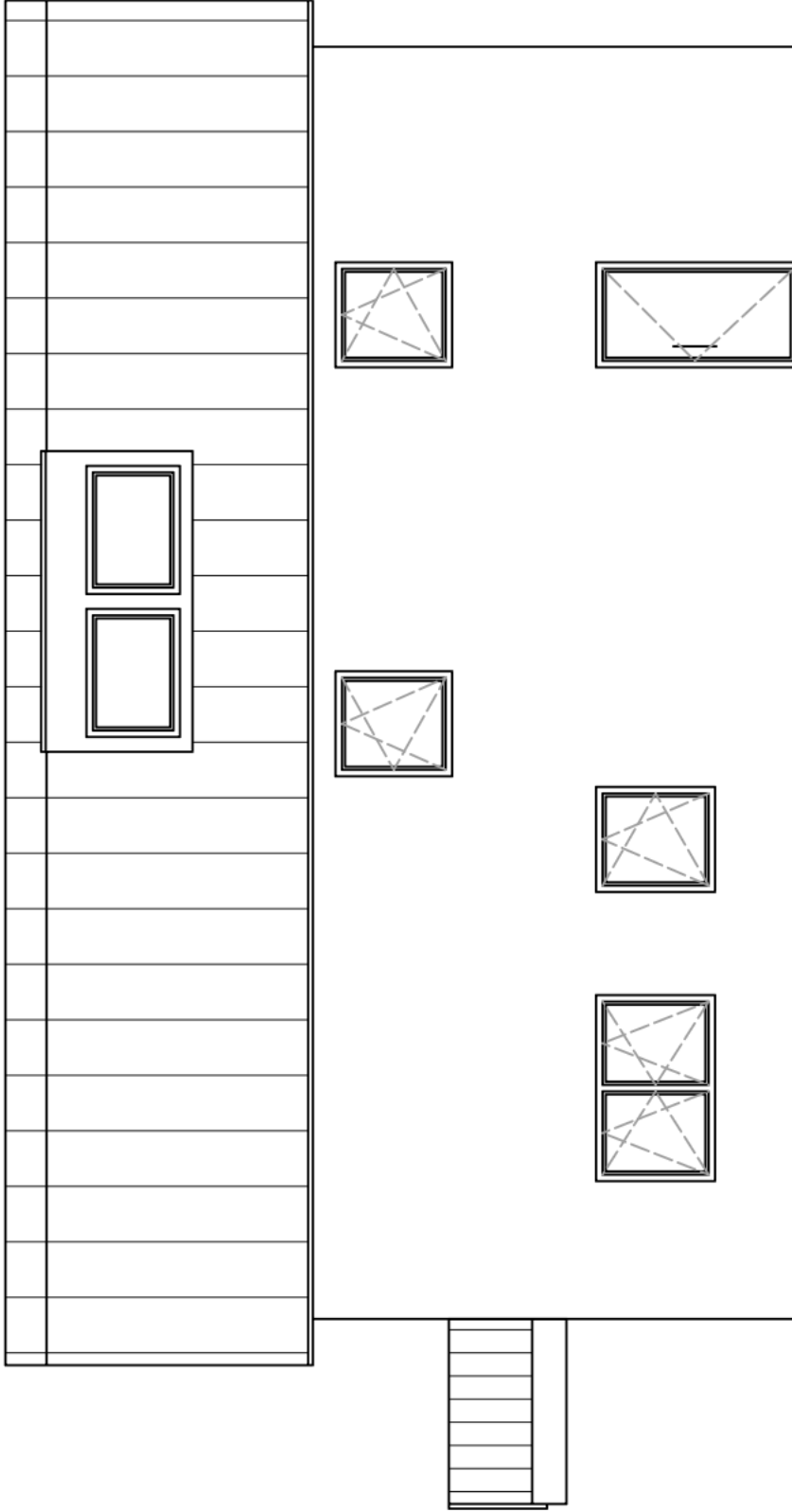
Ansicht Osten
