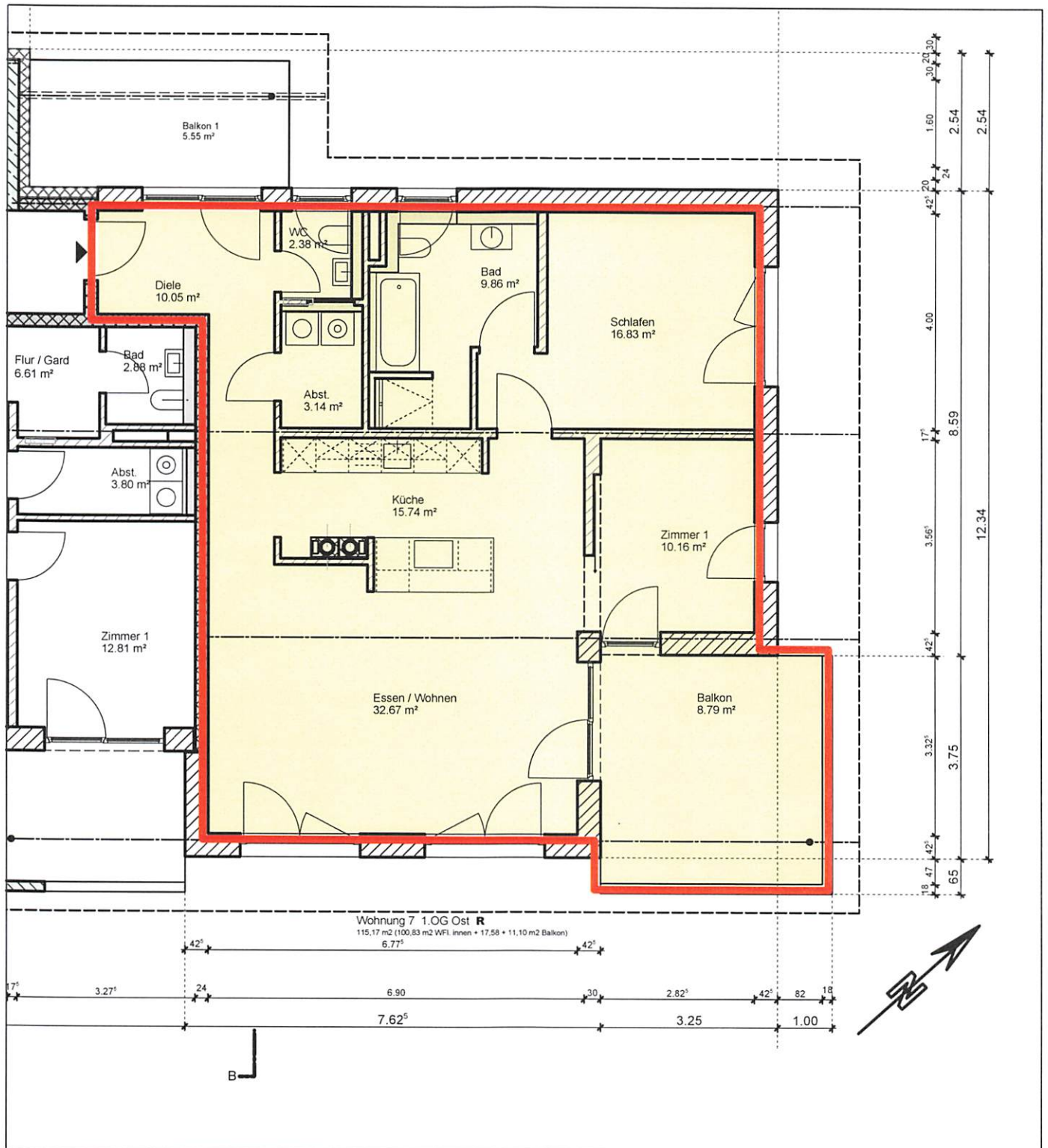
Obergeschoss
