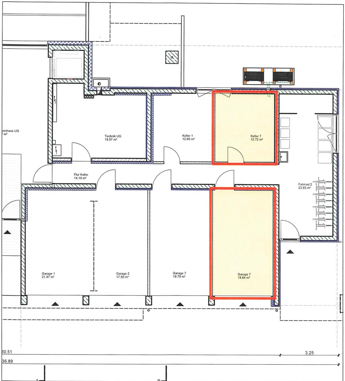
Untergeschoss/Eingangsgeschoss
