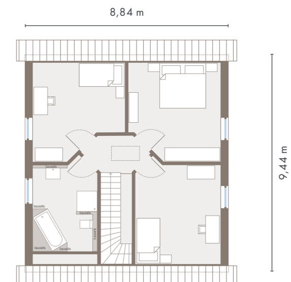
Dachgeschoss 65,28 m 2
