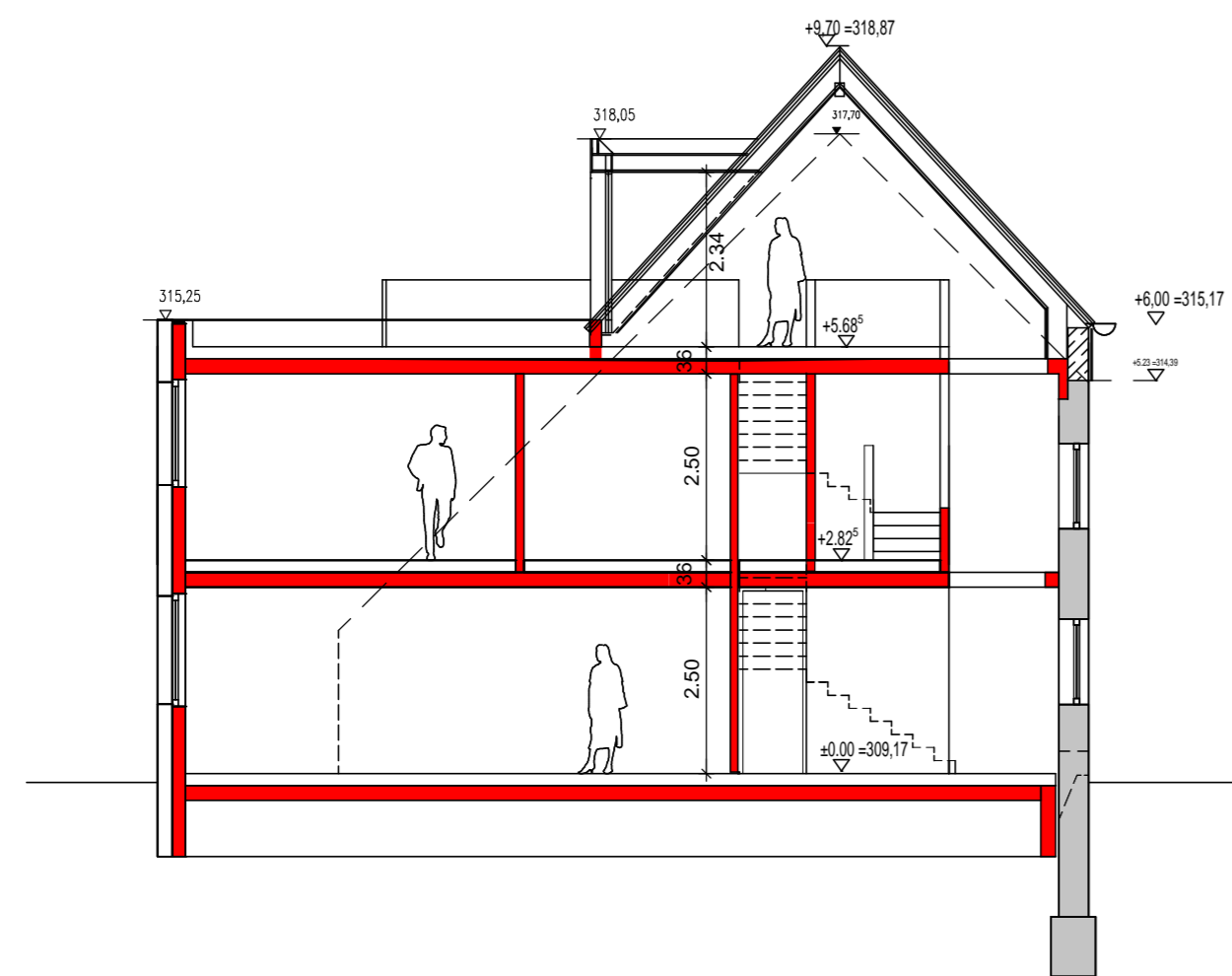
Schnitt AA
