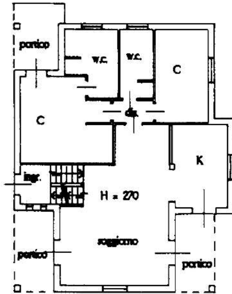
PIANO RIALZATO
