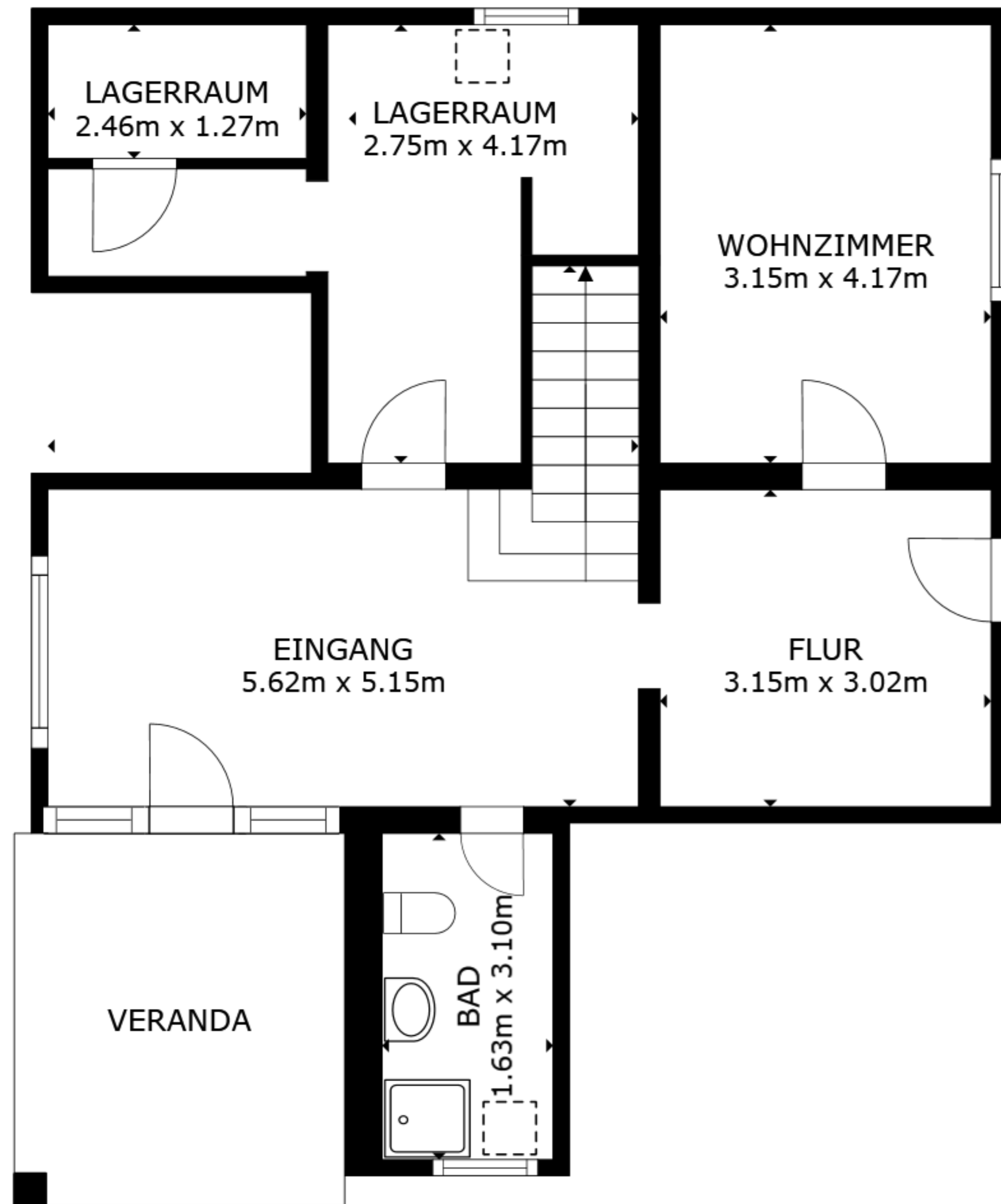
STOCKWERK 1
