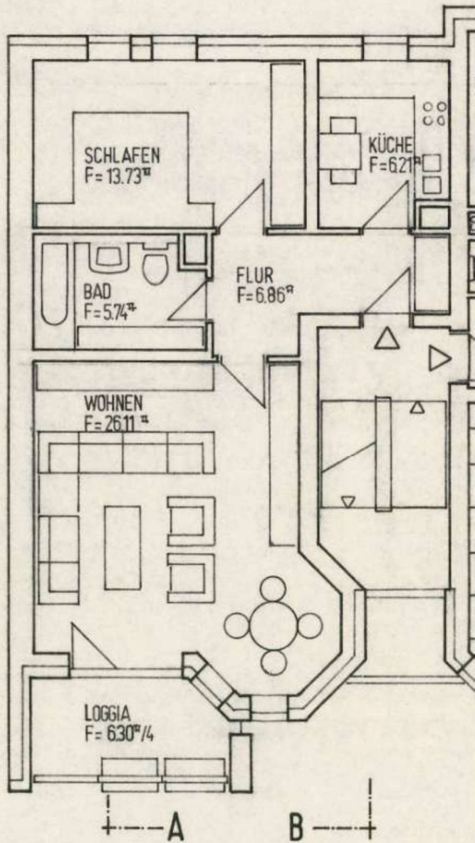
WOHNUNG 4-6
