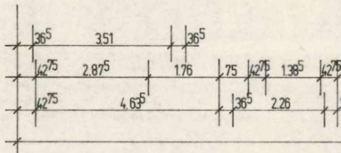
NORMALGESCHOSS
