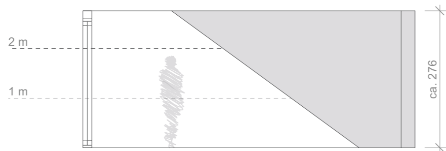
SCHEMATISCHER SCHNITT
