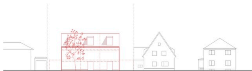
Ansicht Süd
